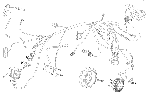
INSTALACIÓN ELÉCTRICA - ELECTRICAL SYSTEM
