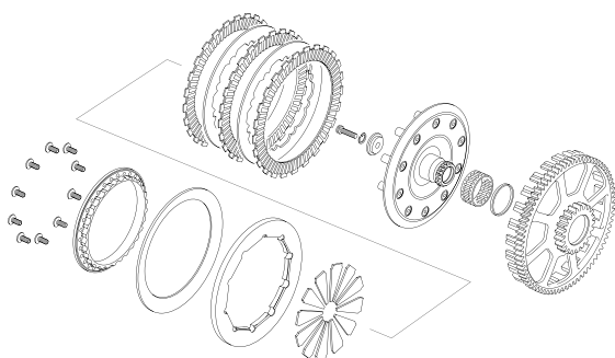
EMBRAGUE - CLUTCH
