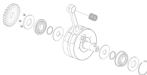
CIGUEÑAL - CRANKSHAFT
