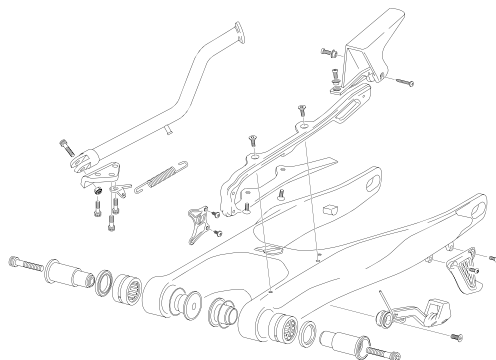
BASCULANTE - SWINGARM
