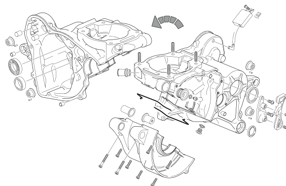
CÁRTERS - CRANKCASE
