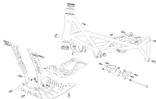
BASTIDOR - FRAME
