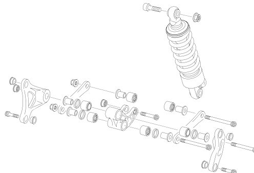
AMORTIGUACIÓN - ROCKER
