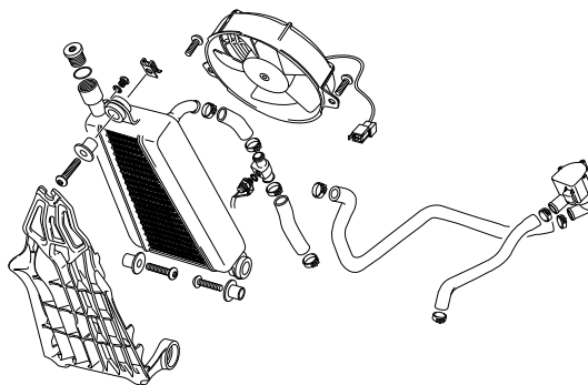
REFRIGERACIÓN - COOLING SYSTEM
