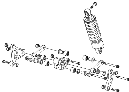
AMORTIGUACIÓN - ROCKER
