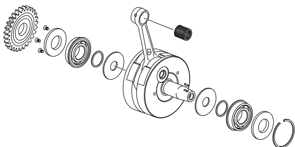
CIGUEÑAL - CRANKSHAFT
