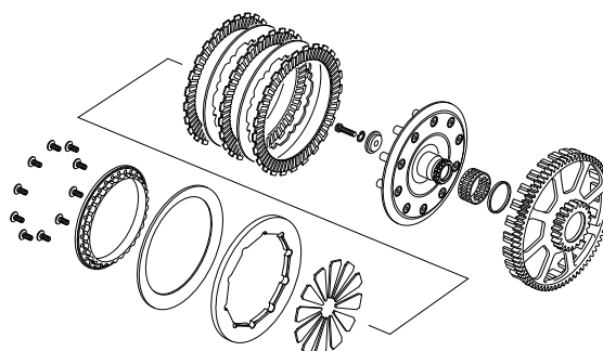
EMBRAGUE - CLUTCH
