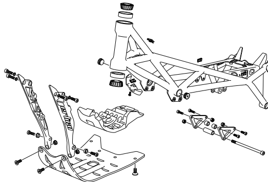
BASTIDOR - FRAME
