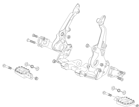
SUBCHASIS - SUBFRAME
