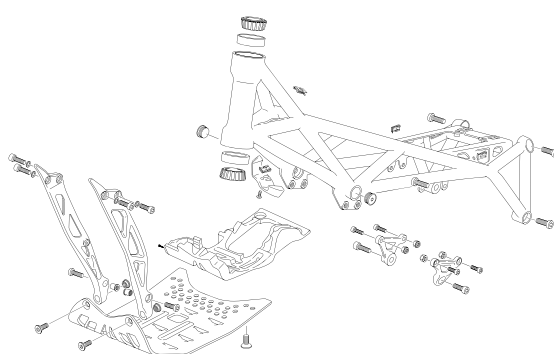
BASTIDOR - FRAME
