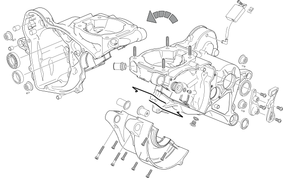
CÁRTERS - CRANKCASE
