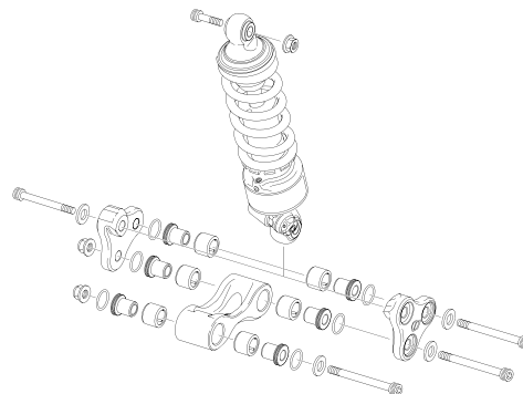
AMORTIGUACIÓN - ROCKER
