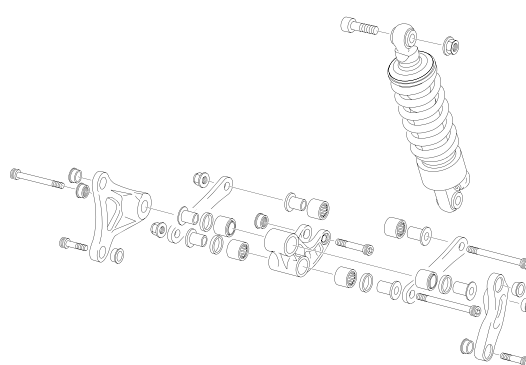
AMORTIGUACIÓN - ROCKER
