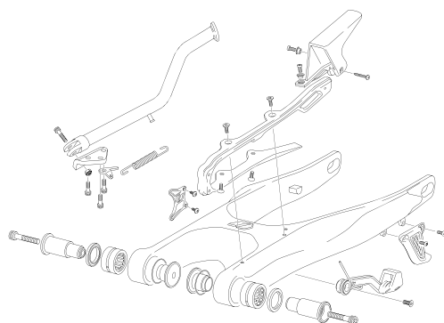
BASCULANTE - SWINGARM
