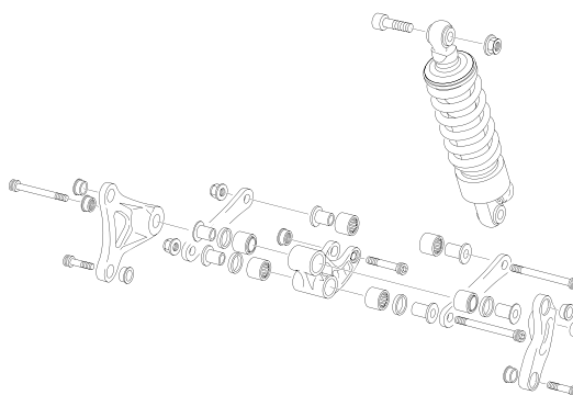
AMORTIGUACIÓN - ROCKER
