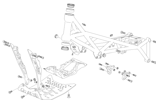
BASTIDOR - FRAME
