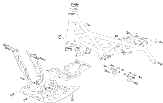
BASTIDOR - FRAME
