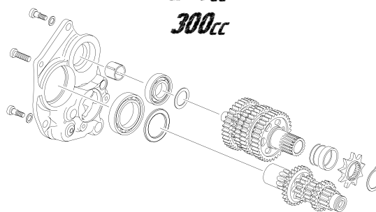
CAMBIO DE MARCHAS - GEARBOX
