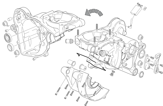
CÁRTERS - CRANKCASE
