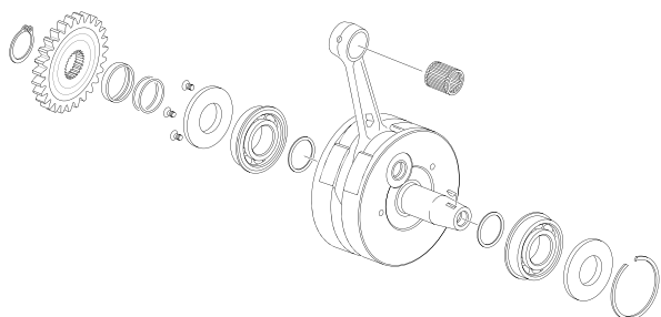
CIGUEÑAL - CRANKSHAFT
