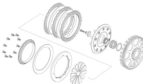
EMBRAGUE - CLUTCH
