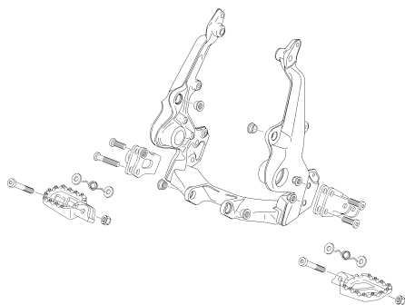
SUBCHASIS - SUBFRAME
