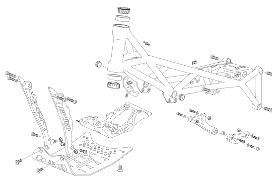
BASTIDOR - FRAME
