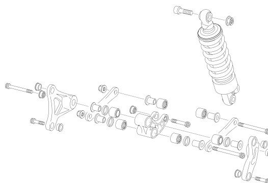
AMORTIGUACIÓN - ROCKER
