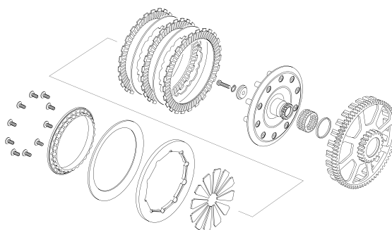
EMBRAGUE - CLUTCH
